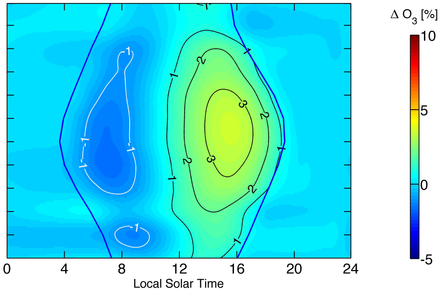
b) WACCM, p=5.76 hPa
