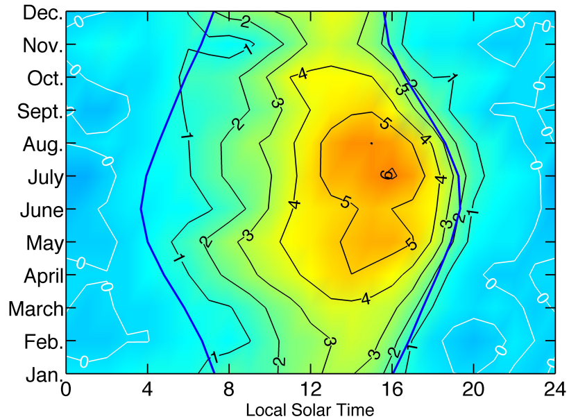
a) GROMOS, p=5.76 hPa
